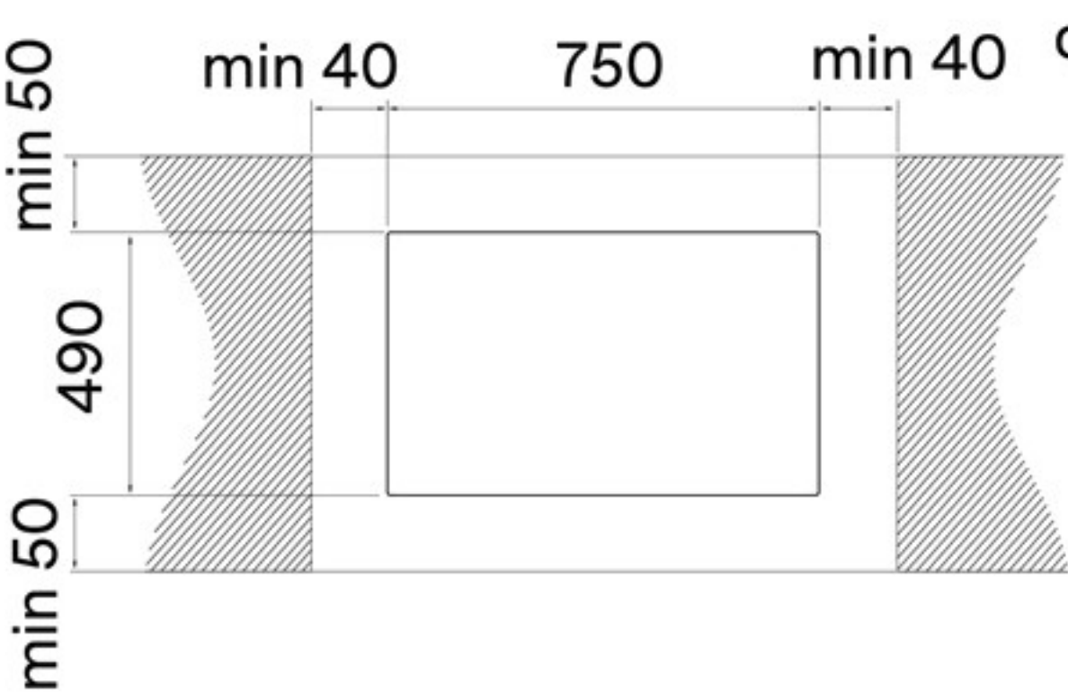
MUNKALAPRA szereelés
